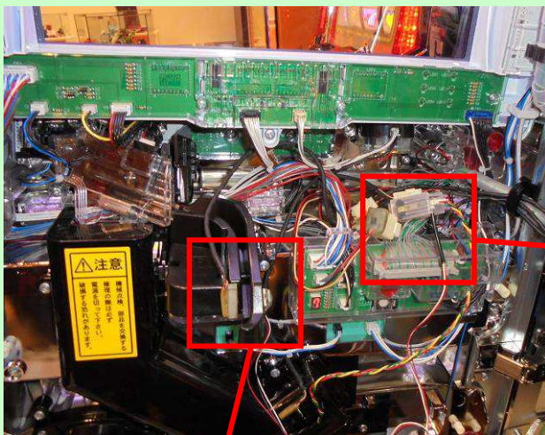
電流センサー取付例
