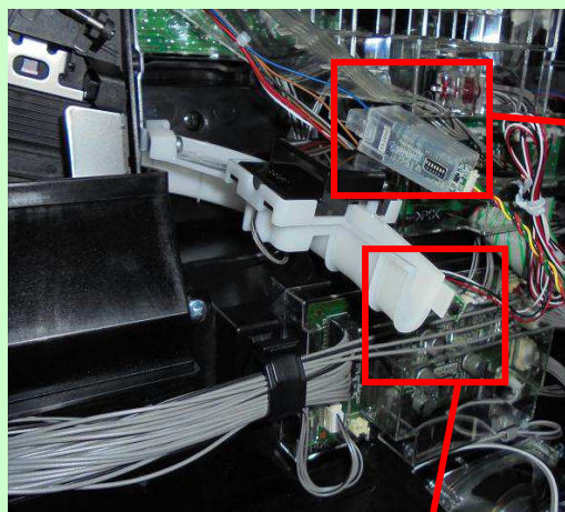
電流センサー取付例
