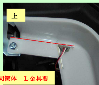
電流センサー取付例
