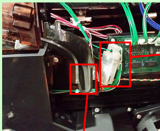
反射センサー取付例
